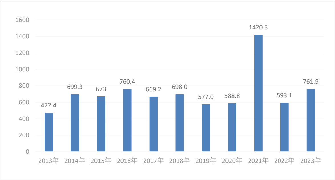
图 1-4 2013-2023 年济源市年降水量柱状图
